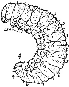
Fig. 354. Euparius marmorius Oliv.
